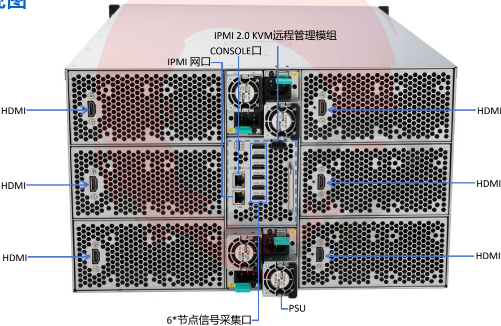
后视图
