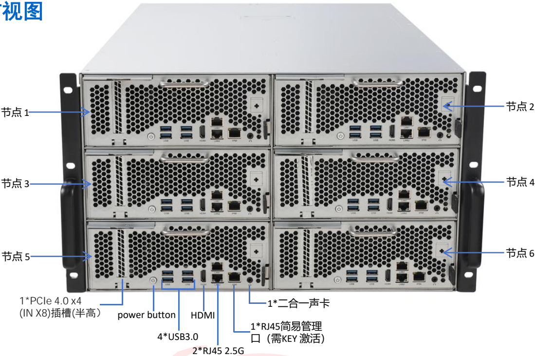
后视图
