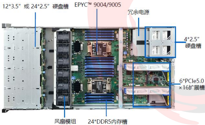
内部构造图
