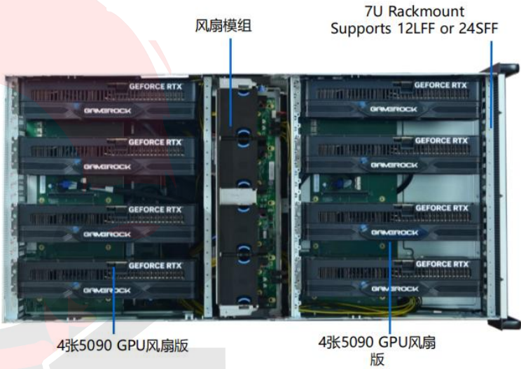
内部构造图
