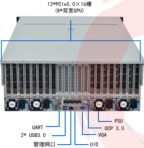
后视图
